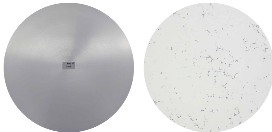
Sezione micrografica d424mm: Area di segregazione 8 mm
